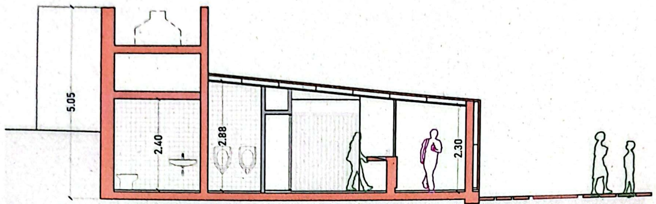
CORTE A-A
