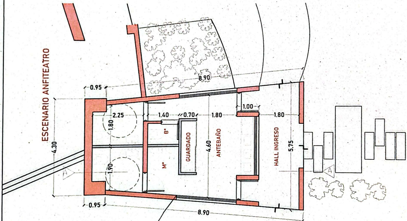
PLANTA GENERAL
